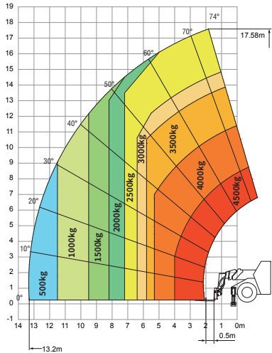
TH45-18 支腿支撑 载荷图
